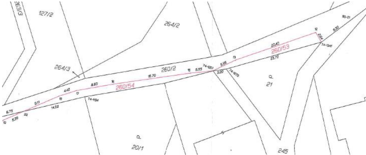
Výřez z Geometrického plánu č. 93-272/2014.
