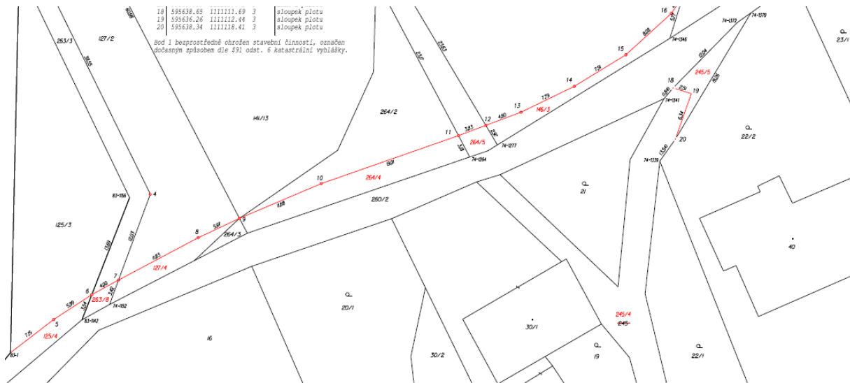
Výřez z Geometrického plánu č. 108-9/2019.
